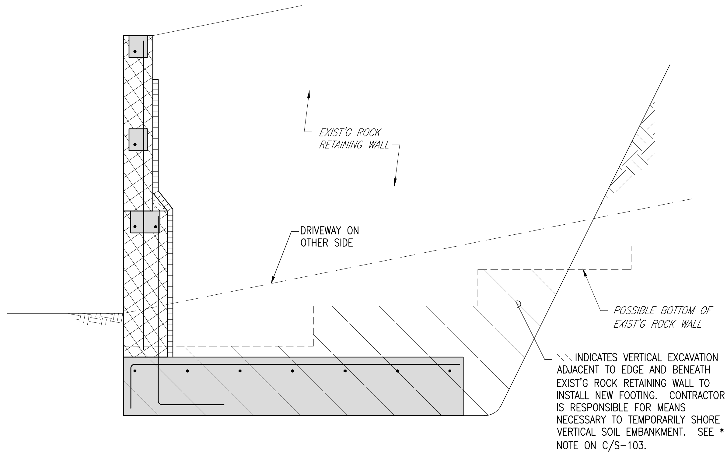
B SECTION S-103 SCALE: NTS
